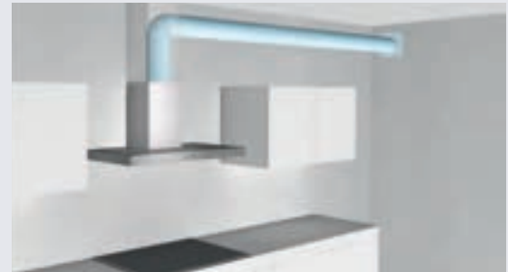
Beispiel einer guten Verrohrung
